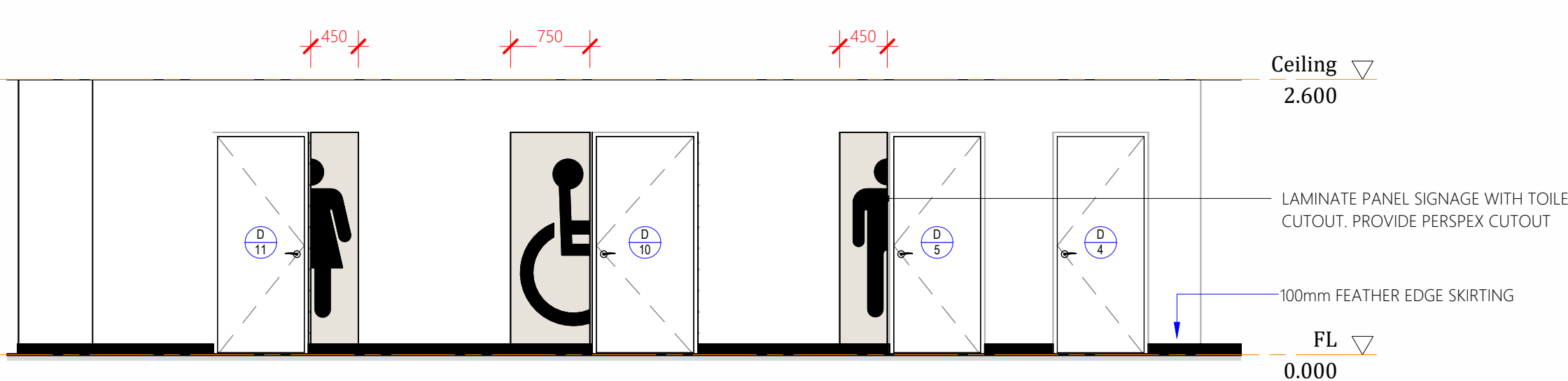
Elevation 2E
