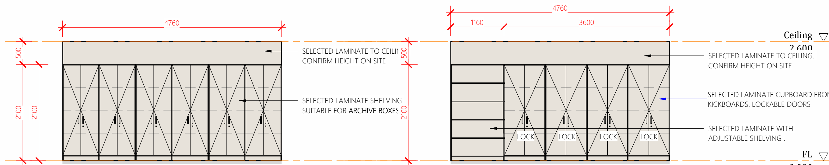
Elevation 2A
