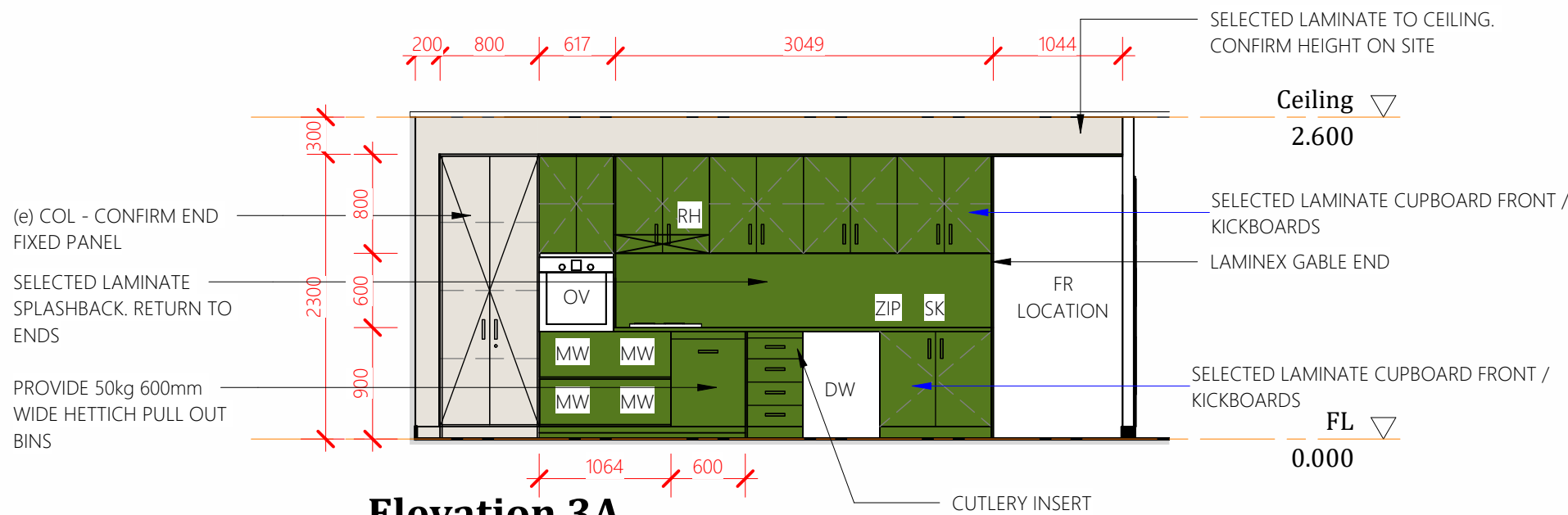
Elevation 3A
